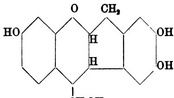
Brasilin
